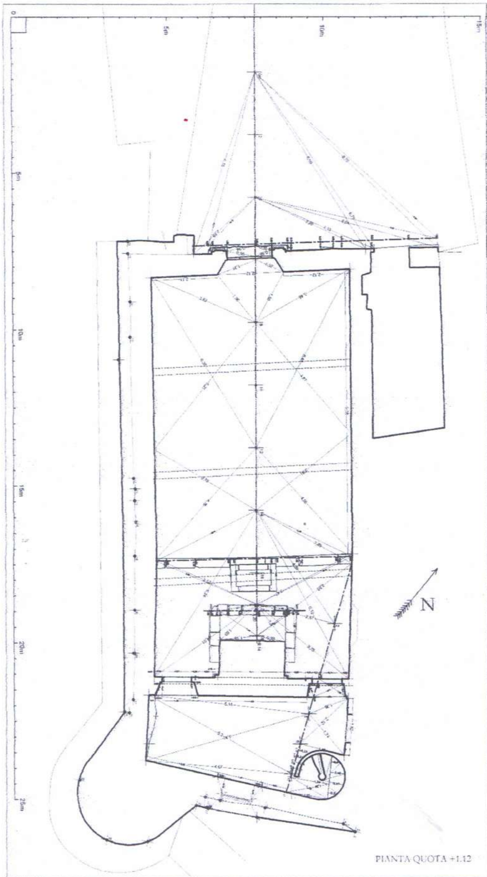
Pianta a livello di ingresso, rilievo geometrico
