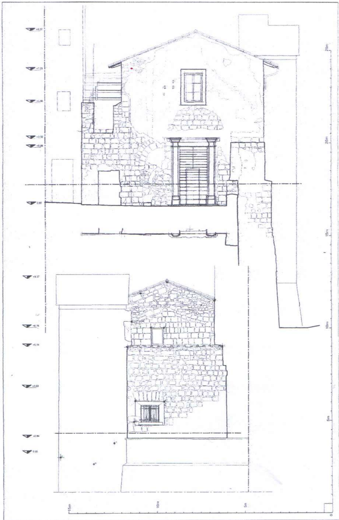
Prospetti nord e sud.
